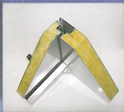
Construction double peau 30 ou 60 mm
